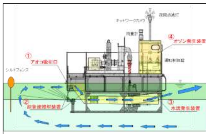
図 36 アオコ抑制装置側面図（寸法：全長 5,200mm × 全幅 3,690mm）
